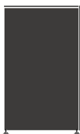
Verbindungsmodul ohne Schloss Wahlweise Anschlag links / rechts H 1200 x B 747 x T 900
